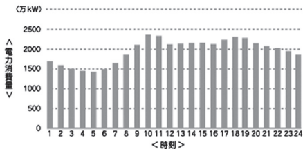
一日の電気の使われ方（冬季の場合）
