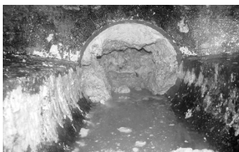
油により閉塞した下水道管
