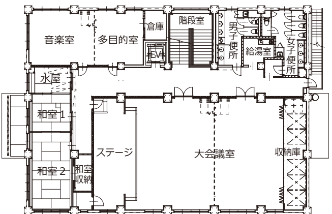
2階平面図
