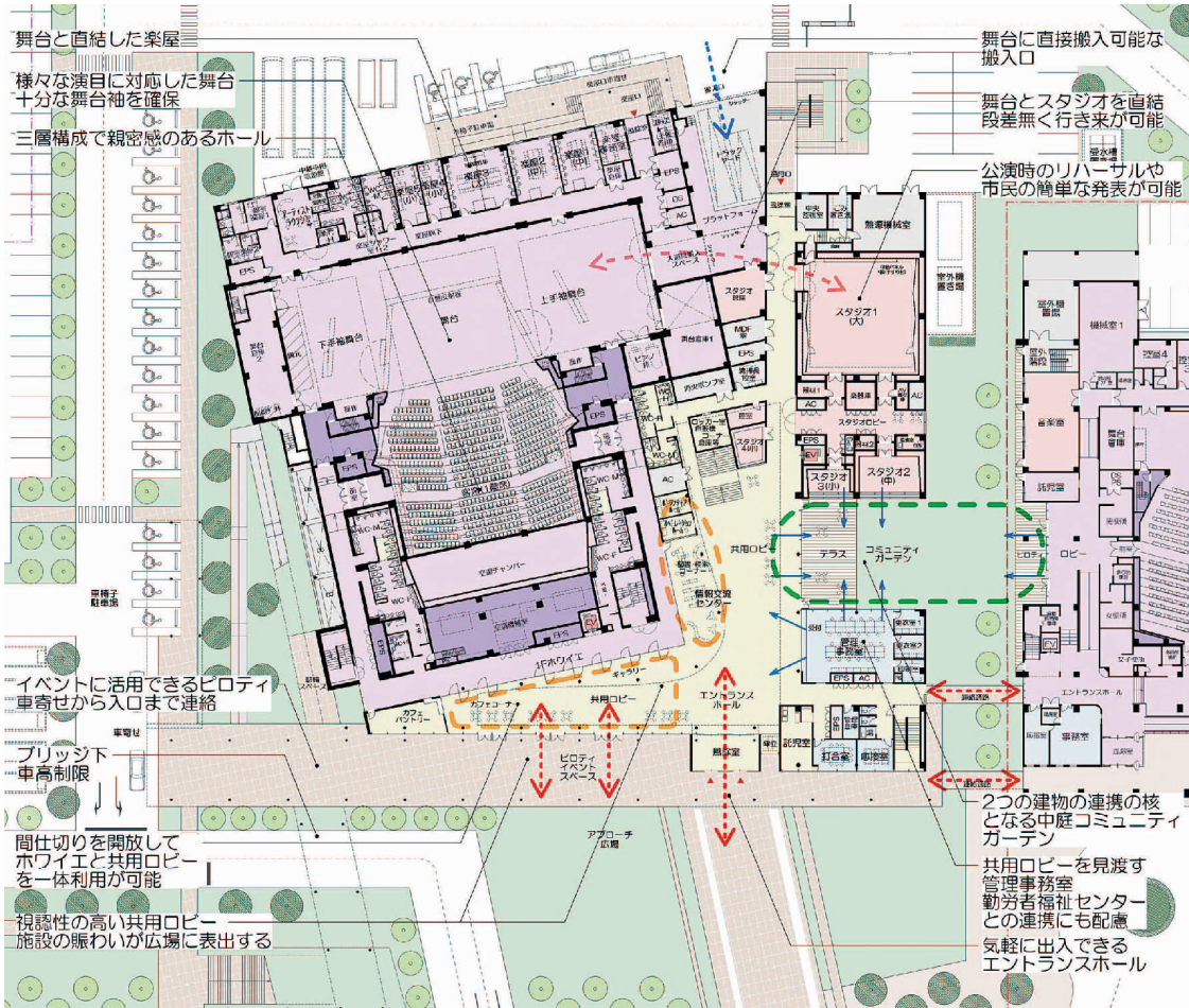
佐久市総合文化会館 平面計画図（基本設計より）
